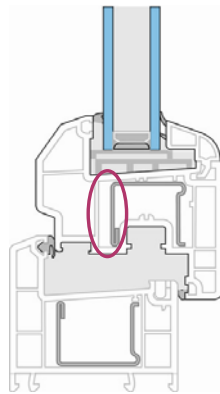
REHAU-Thermo-Block: zusätzliche isolierende Luftkammer
